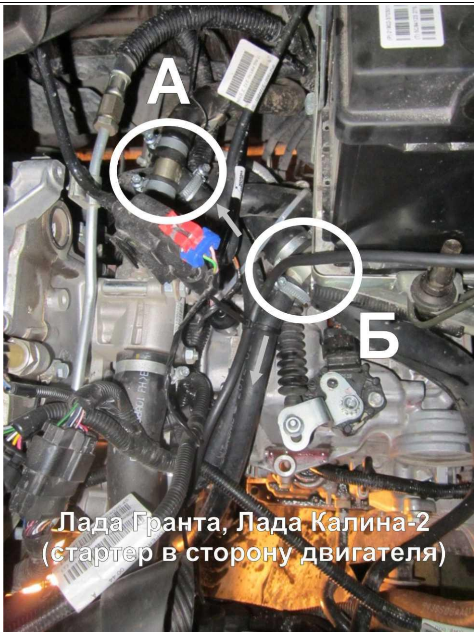
Рис. 4. Врезка тройников на Гранту и Калину-2. Вид сверху
