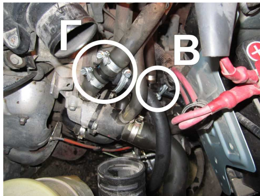
Рисунок 5. Тройник входного рукава В. Тройник выходного рукава Г. Вид сверху.
